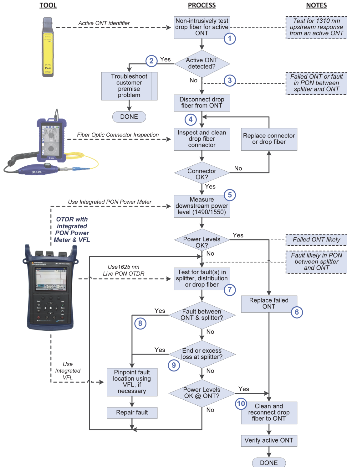
Fig. 4— Troubleshooting a Live PON
